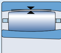
Радиальный внутренний зазор подшипников CARB с коническим отверстием
