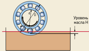
Уровень масла в масляной ванне
